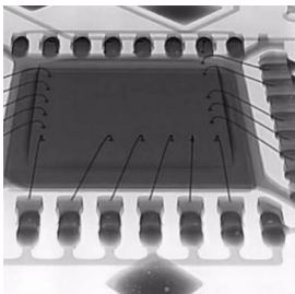
IC WIRE
