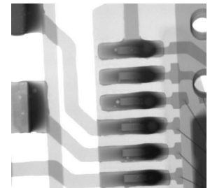
IC Soldering
